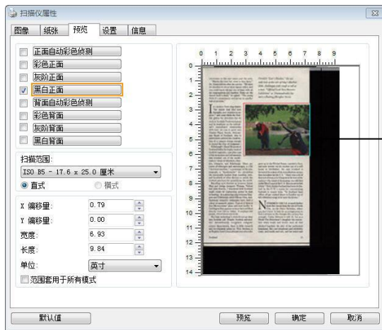
「预览」页签
